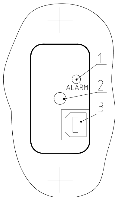
Рисунок 1.3 – Органы настройки блока ПРМ-ПРД извещателей «ЗЕБРА-30(24)-О»
